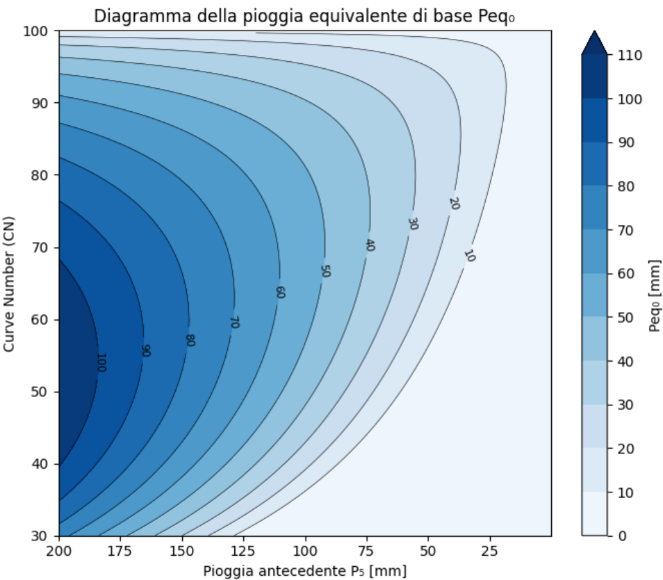
Metodo delle piogge equivalenti: pioggia equivalente di base P_{eq0} in funzione del numero di curva CN e della pioggia antecedente P_5
