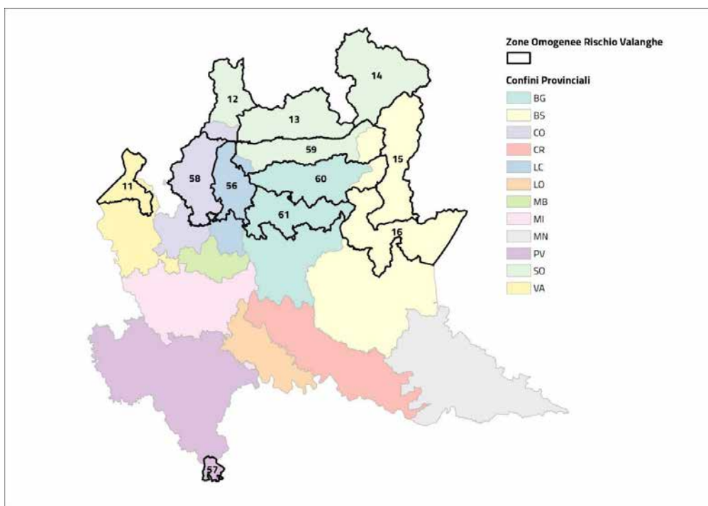
Zone omogenee per rischio Valanghe
