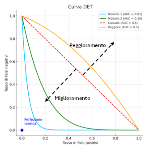
Curva DET
