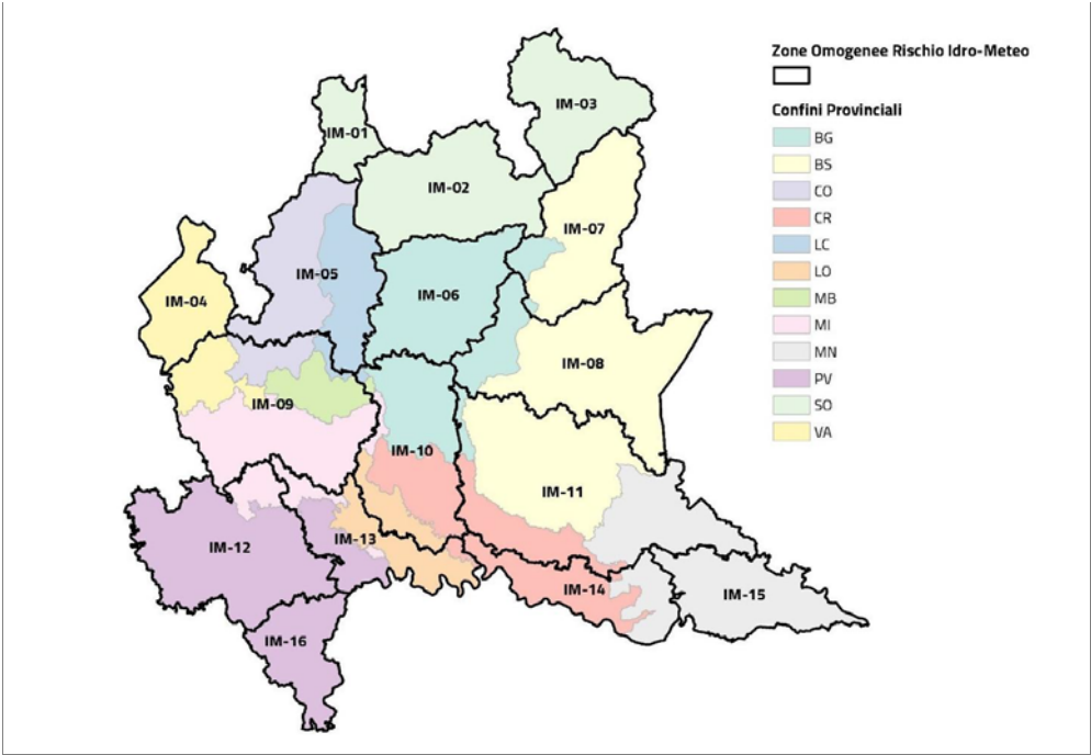
Zone omogenee per rischio Idro-Meteo
